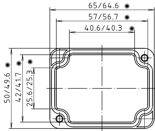
Deckel / lid
