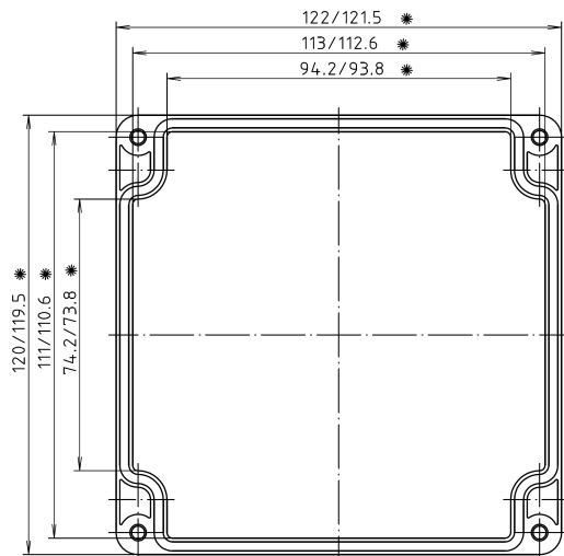
Deckel / lid
