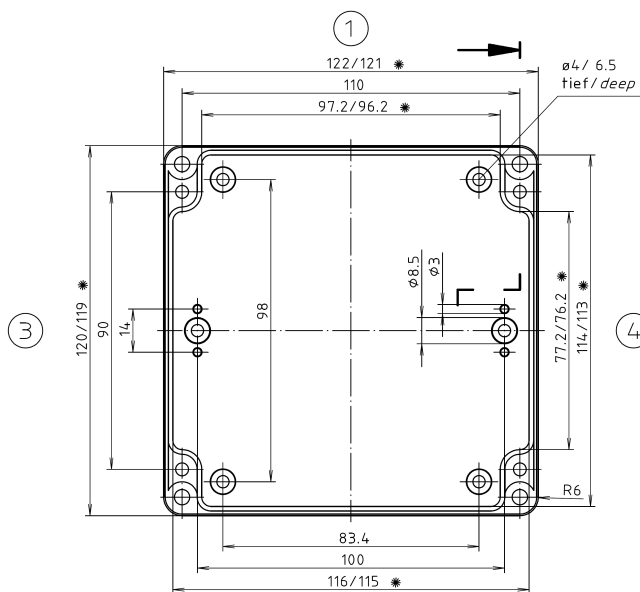
Unterteil / base
