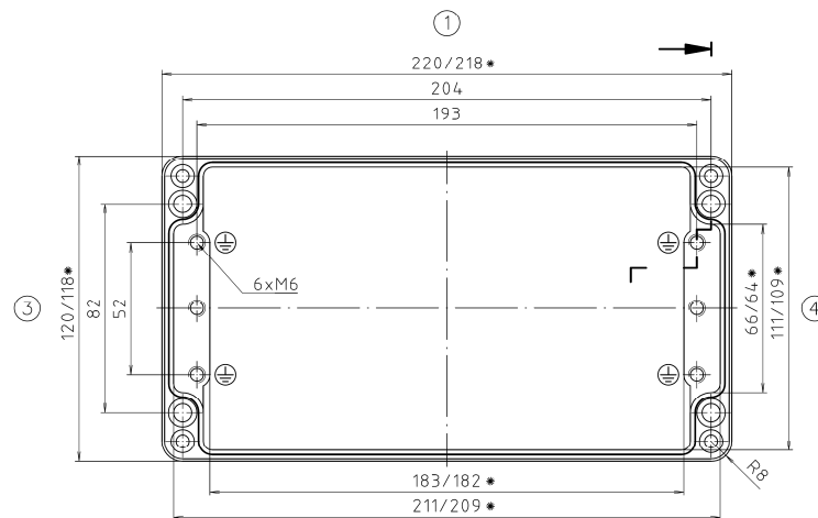
Unterteil / base
