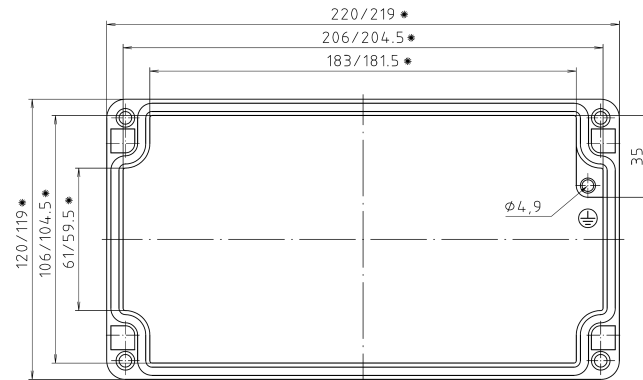
Deckel / lid
