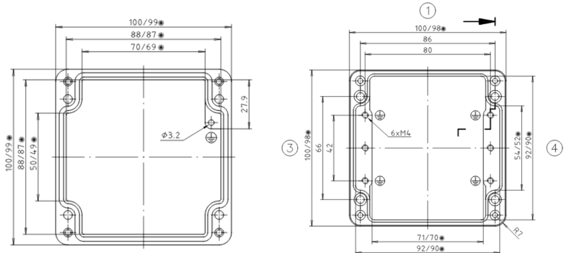
Deckel/ lid
